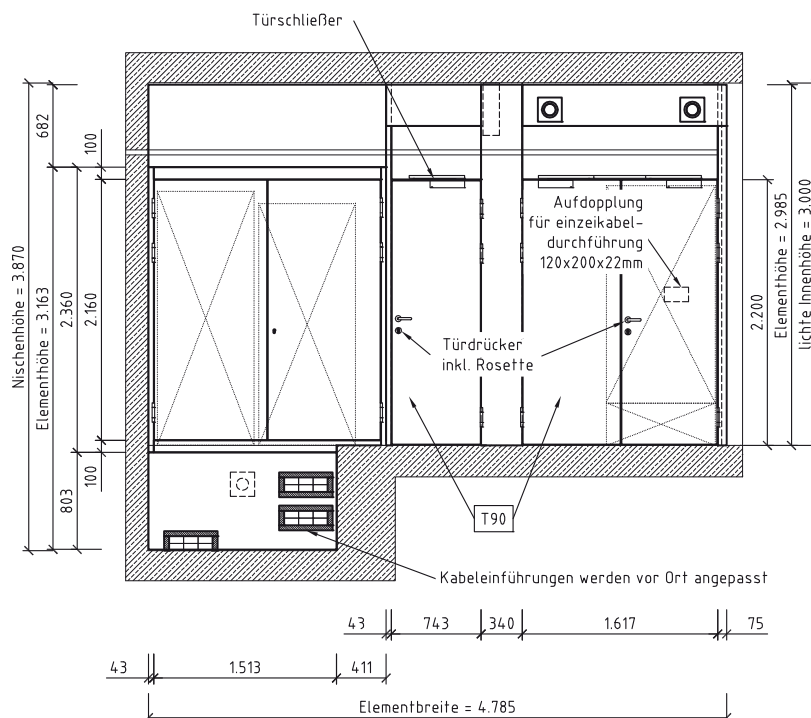
Vorderansicht
