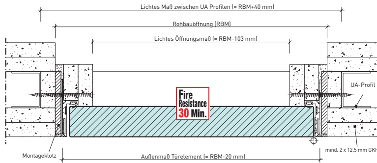
Einbau PRIODOOR ETX A in Schachtwand GKF, beidseitig beplankt
