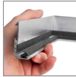
■ Zweistufiges Dichtungssystem: heiß- und kaltrauchdicht
