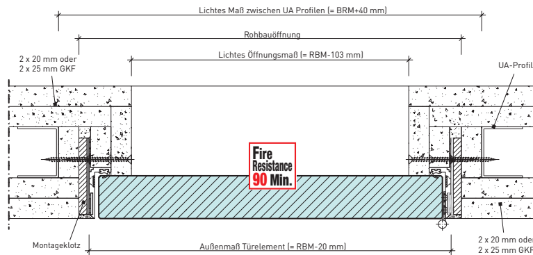
Einbau PRIODOOR ETX A in Schachtwand GKF, beidseitig beplankt
