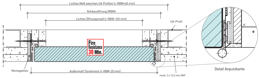
Einbau PRIODOOR ETX A in Schachtwand GKF, einseitig beplankt
