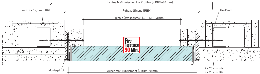
Einbau PRIODOOR ETX A in Schachtwand GKF, einseitig beplankt
