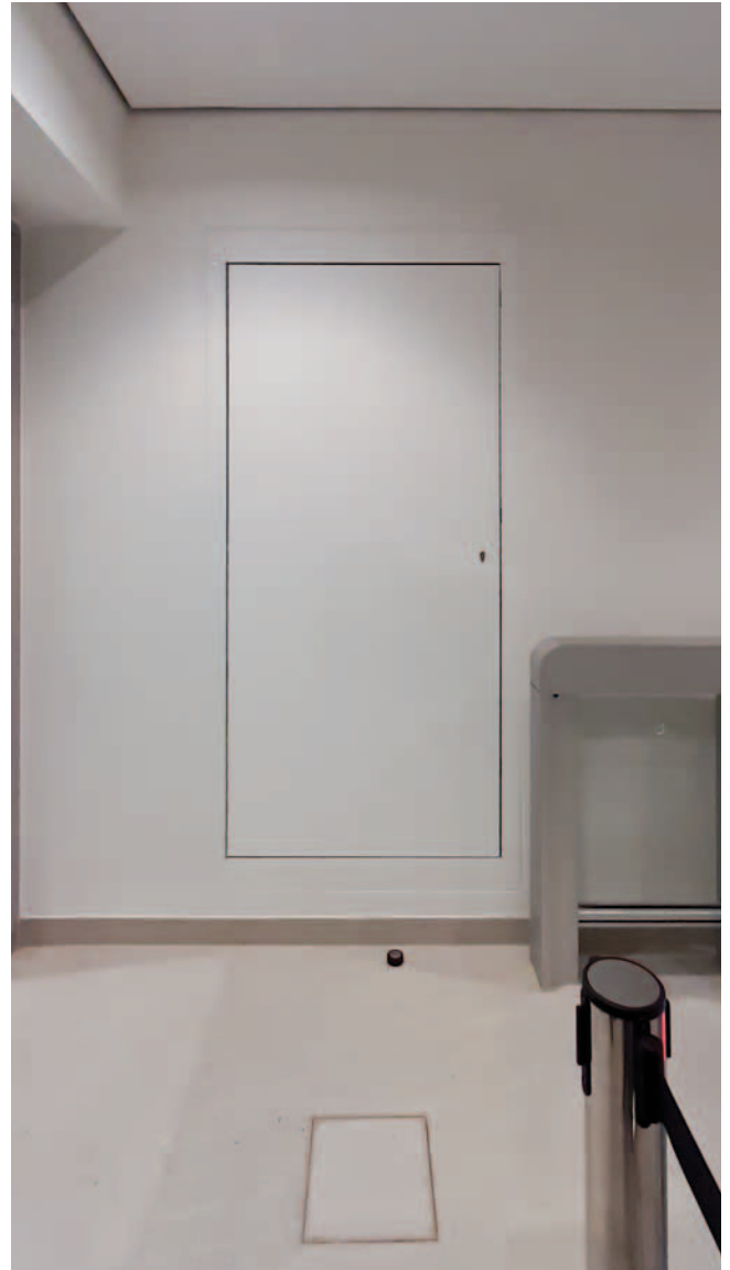
Feuerwiderstandsfähige Abtrennung der Installationsschächte mit PRIODOOR RTH
